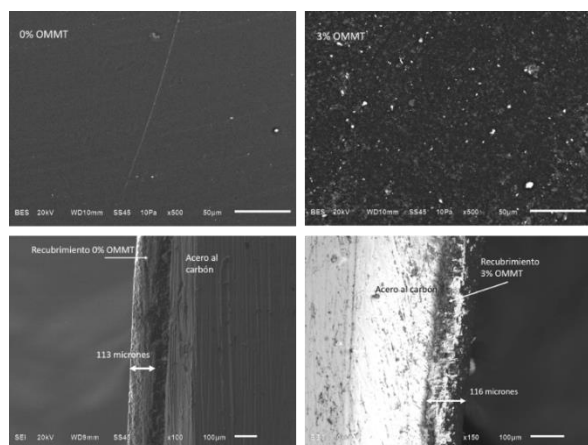
Figura 1. Imágenes de SEM de la superficie de los recubrimientos: (a) 0 % OMMT, (b) 3 % OMMT; sección transversal de los recubrimientos, (c) 0 % OMMT, (d) 3 % OMMT.
