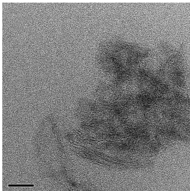
Figura 2. Imagen de TEM de la muestra 3 % OMMT
