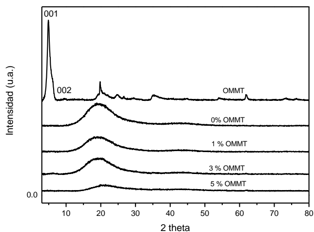
Figura 3. Difractogramas de las muestras OMMT, 0 % OMMT, 1 % OMMT, 3 % OMMT y 5 % OMMT.
