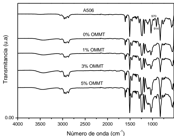
Figura 4. Espectros de FTIR de las muestras A506, 0 % OMMT, 1 % OMMT, 3 % OMMT y 5 % OMMT.
