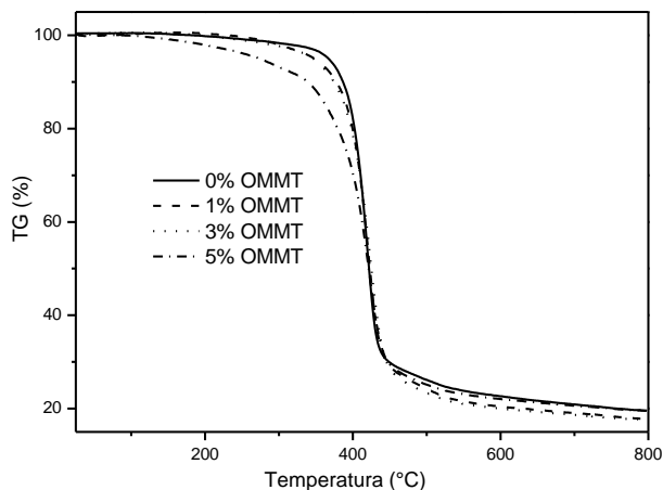
Figura 5. Termogramas de las muestras 0 % OMMT, 1 % OMMT, 3 % OMMT y 5 % OMMT.
